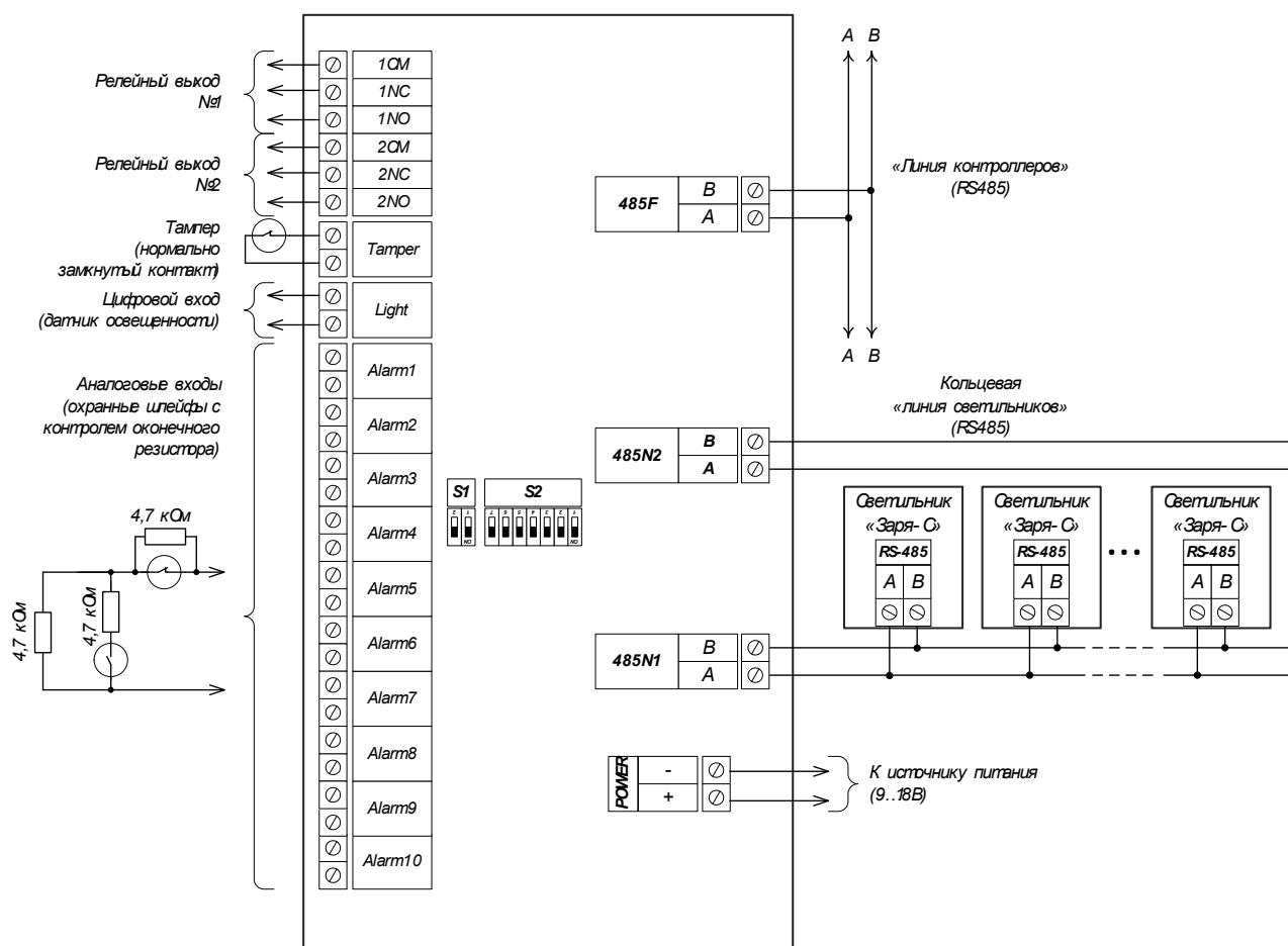
Рисунок 5. Схема подключения контроллера «КЛ-Контур-С»
